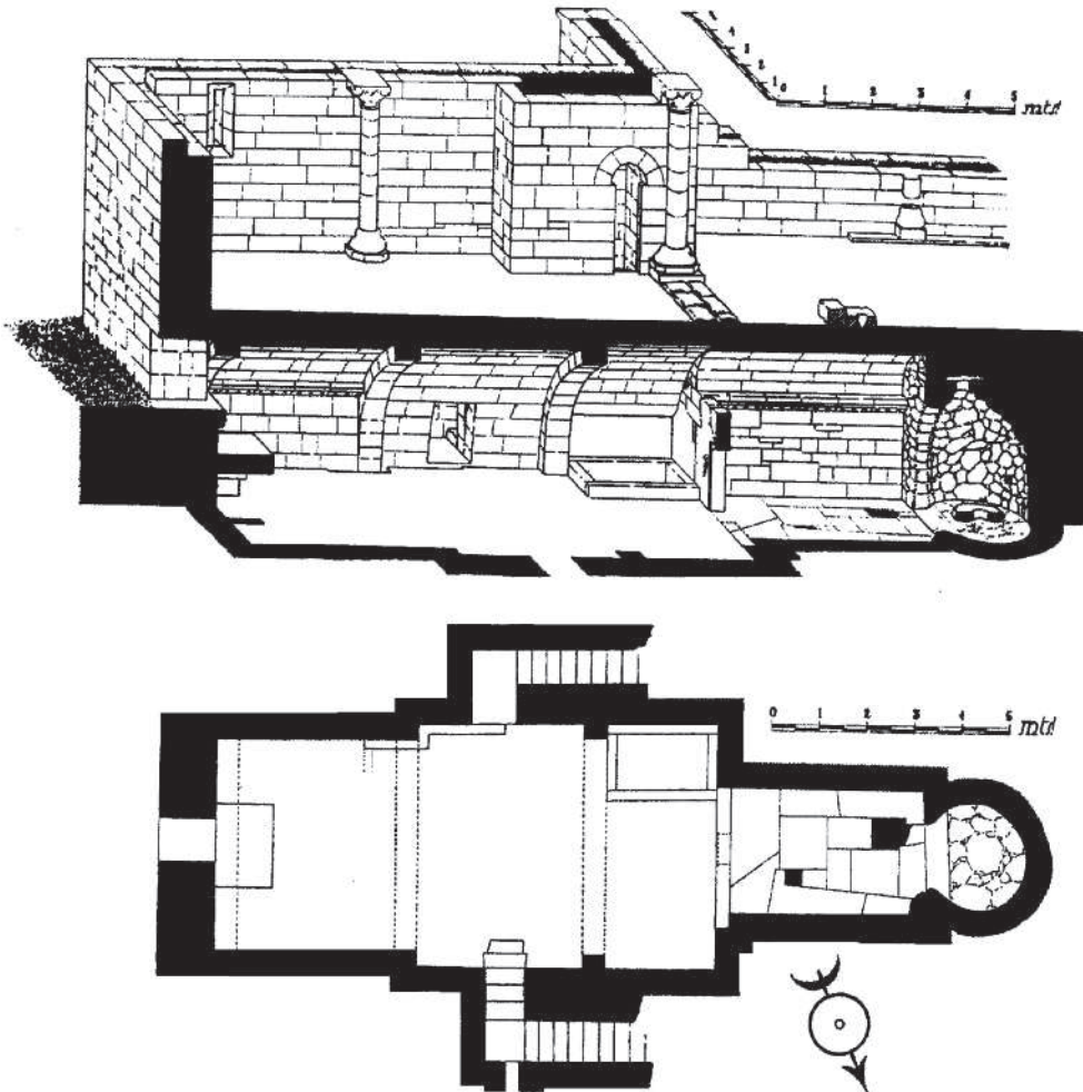
Figura 2. Alzado y planta de Santa Marina de Aguas Santas, con el laconicum (1) y el pilón (2) de la sauna lusitano-galaica.
